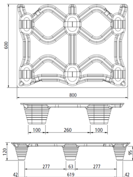
Rozměry INKA palety:
