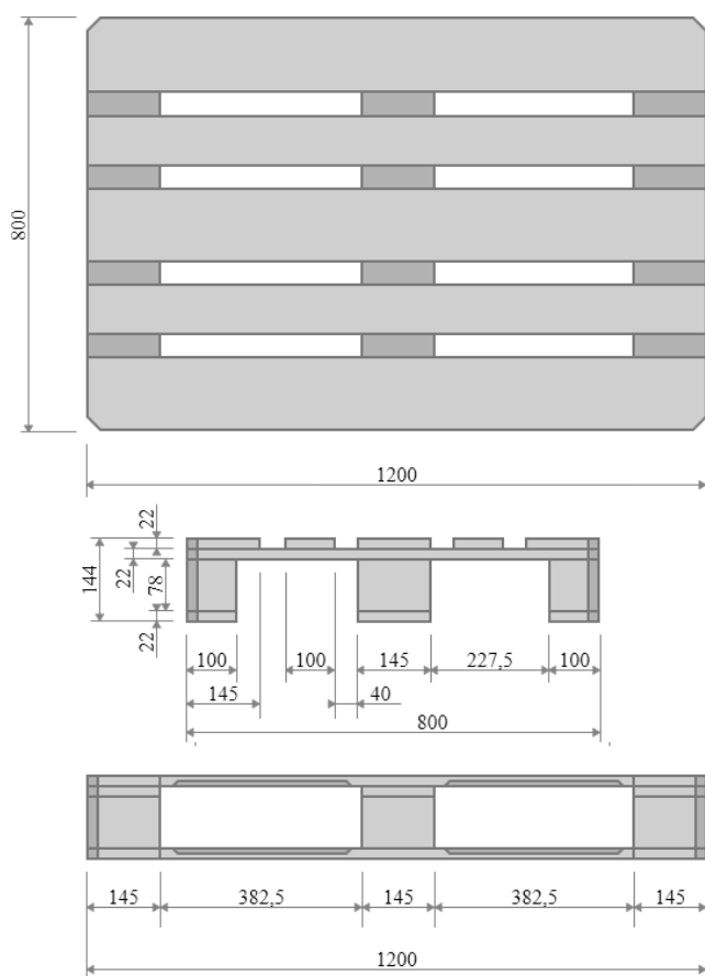
Rozměry EURO palety:
