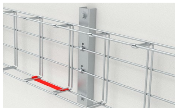
▲▲ Montáž na stojnu pro prostorově vedené kabelové trasy, nebo pro sdruženou nástěnnou montáž více kabelových tras nad sebou.
