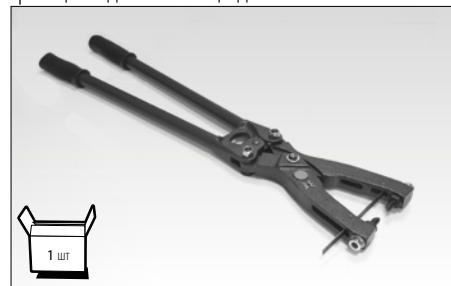
трапецевидные ножницы для системы M2 большие
