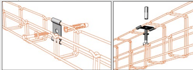
демонстрация монтажа
