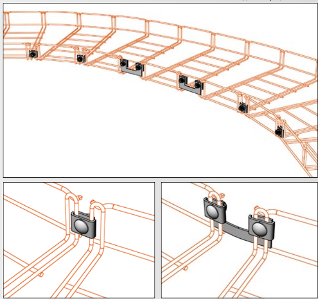
демонстрация монтажа
