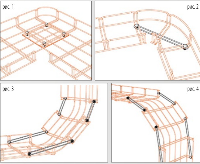
демонстрация монтажа
