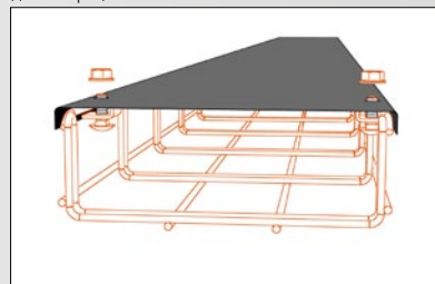
демонстрация монтажа
