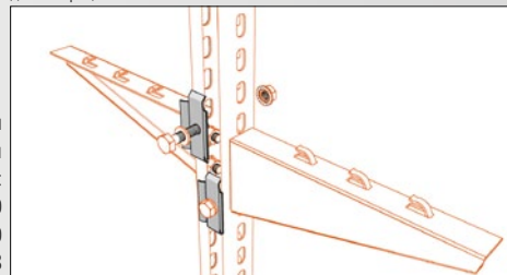
демонстрация монтажа
